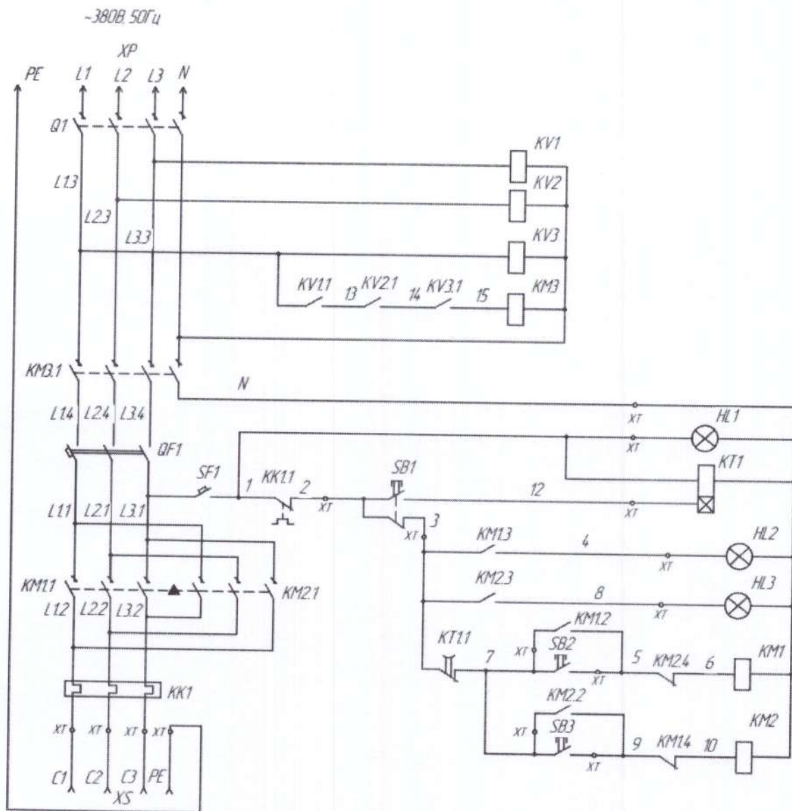
Схема электрическая принципиальная для ПУ
