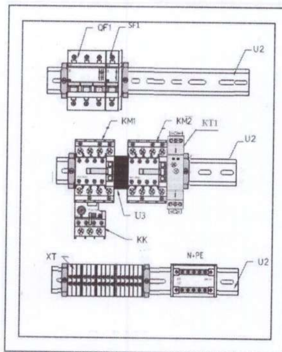
Схема щита управления для ДЭ БУ
